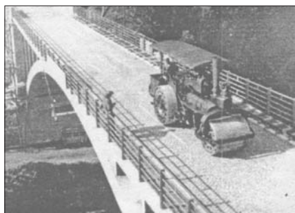
Viadukt při zatěžkávací zkoušce v září 1934
